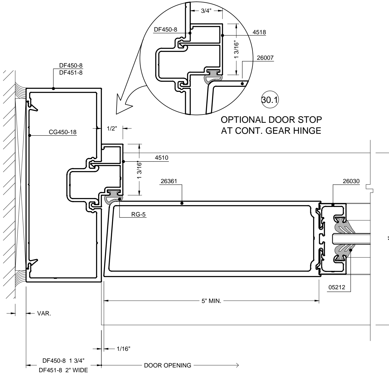
30 WS DOOR JAMB (STANDARD) OFFSET PIVOT & BUTT HINGE
