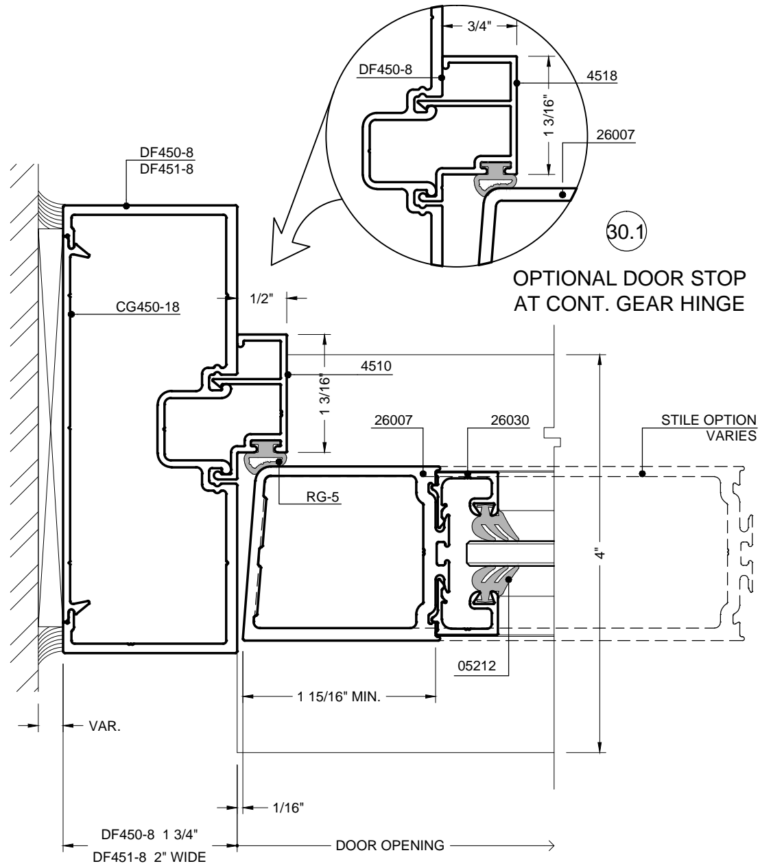
30 DOOR JAMB (STANDARD) OFFSET PIVOT & BUTT HINGE
